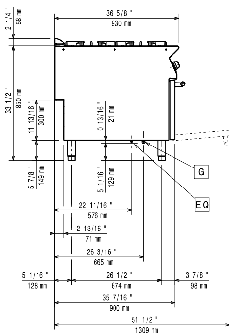
Oldalnézet
